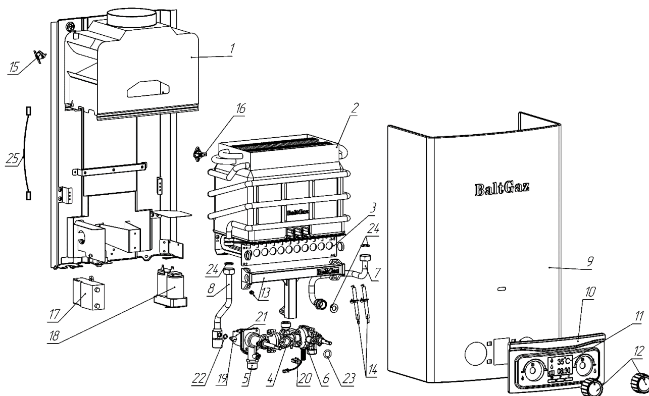
Рисунок 12. Вид аппарата с разнесёнными частями
