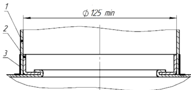
1 – газоотводящая труба; 2 – патрубок газоотводящего устройства аппарата 3 – скотч алюминиевый термостойкий.
