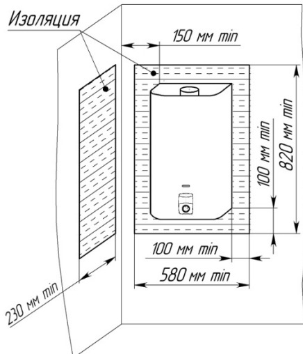
Рисунок 5. Установка аппарата на трудногорюемых стенах
